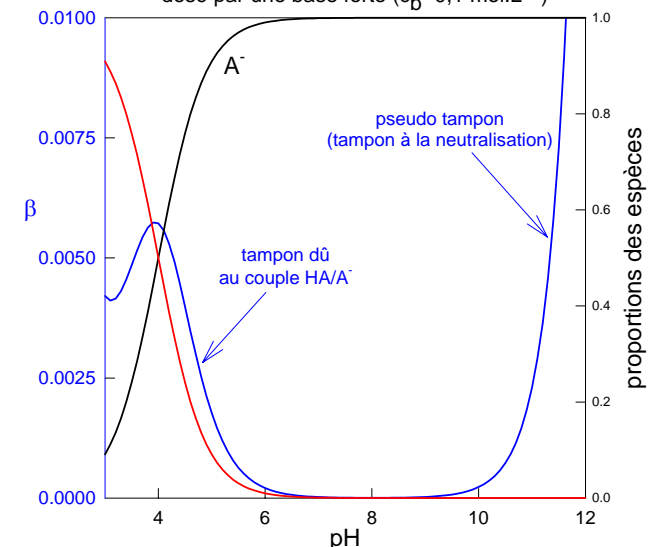
Figure 2 pouvoir tampon et proportion des espèces en fonction du pH d'une solution d'acide faible ( pK_a=6, c_a=0,01 \text{ mol.L}^{-1} ) dosé par une base forte ( c_b=0,1 \text{ mol.L}^{-1} )
